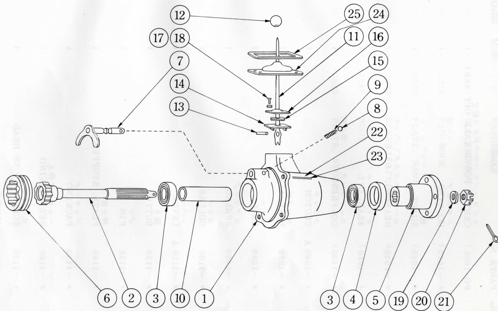
SPC-18H センター・パワー・テークオフ CENTER POWER TAKE OFF
