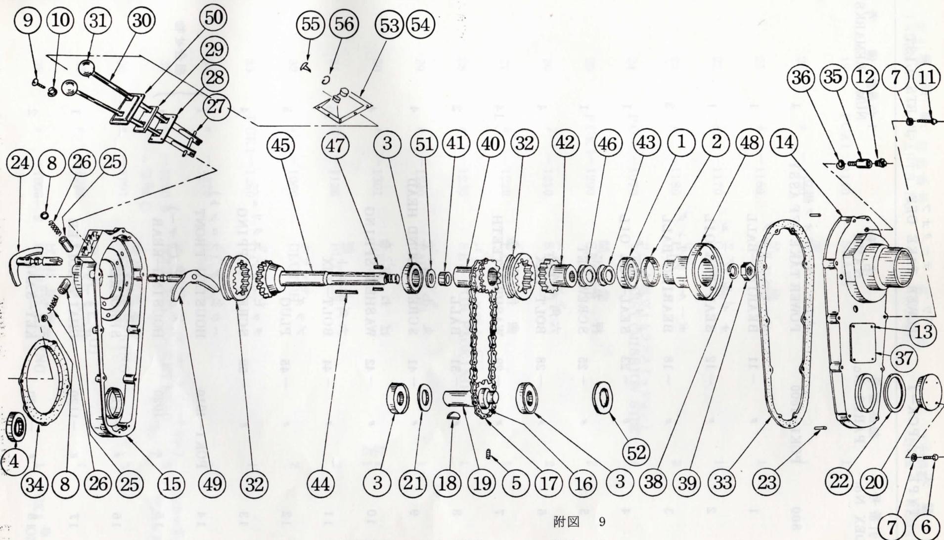
PCK1 パワーテークオフ POWER TAKE OFF
