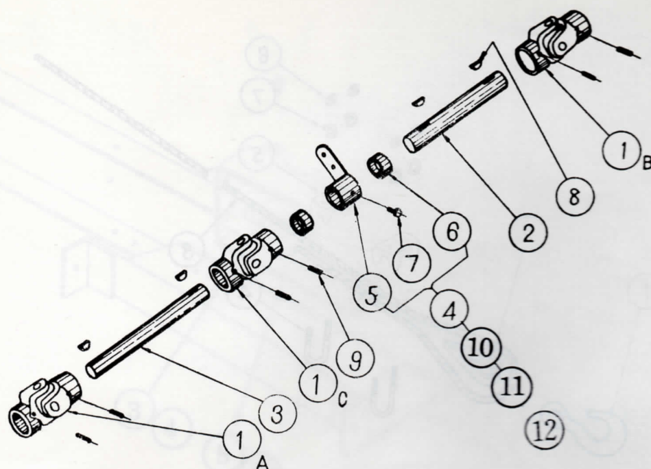
700 ドライブシャフト DRIVE SHAFT
